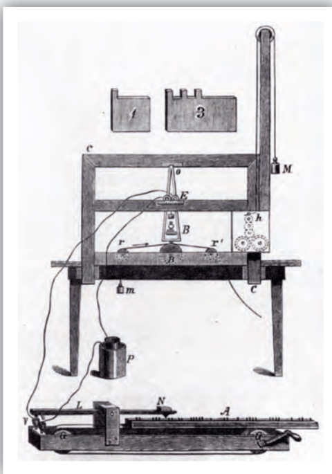
El instrumento telegráfico pendular de Morse, de 1837. El transmisor se ve en la parte inferior.
