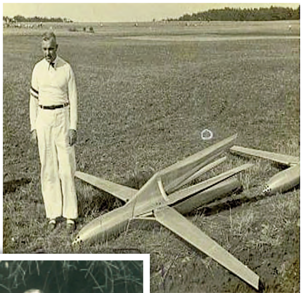
Ingeniero alemán Reinhold Tiling y sus cohetes en 1931.
